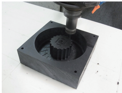
真空注型
