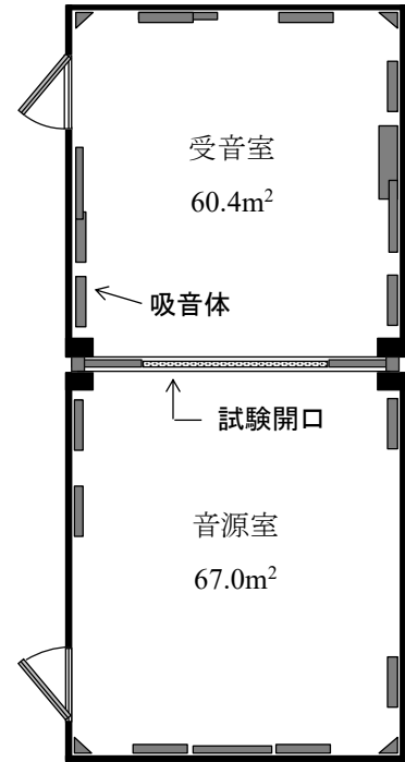
図1 試験室の平面図
