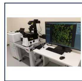
共焦点レーザー顕微鏡
