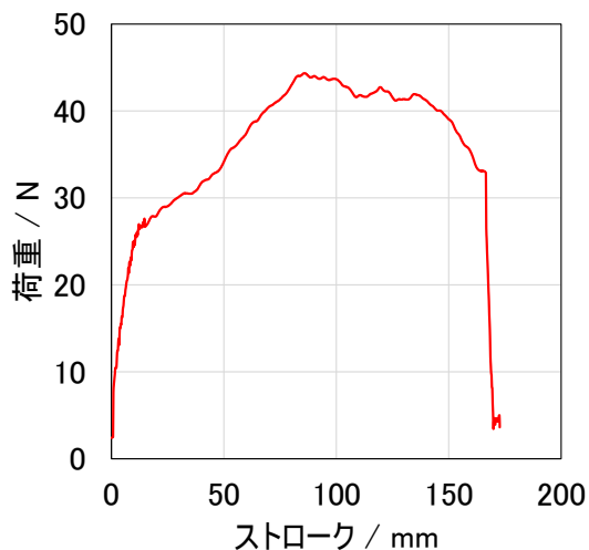
図 2 荷重-ストローク線図
