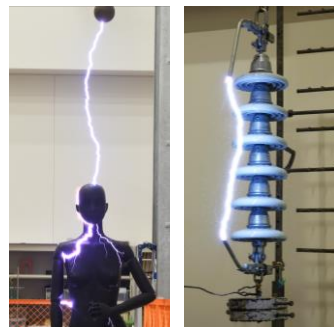
図1 (左) マネキンへの落雷試験
